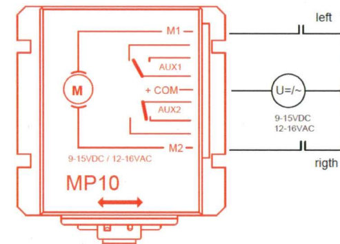
3 wire schematic MP1, MP4, MP8, MP10
