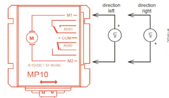
2 wire schematic MP4, MP10
